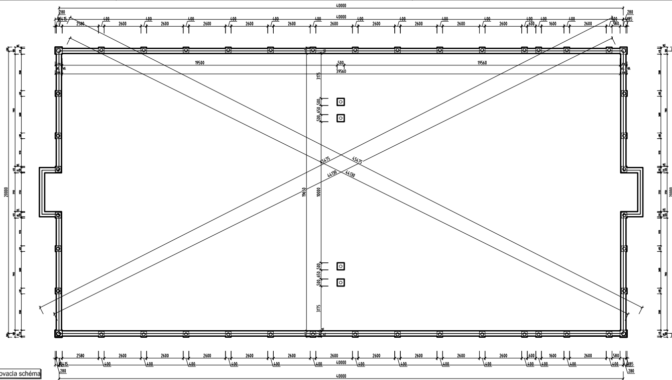
Vytýčovací schéma M 1:50
